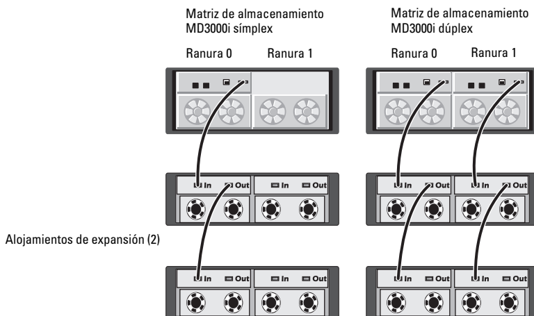
Figura 1. Matriz de almacenamiento RAID MD3000i símplex frente a dúplex (con expansión)
